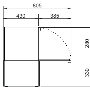
VISTA LATERAL (PORTA ABERTA)
